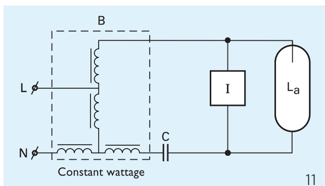
Schéma de câblage 11
