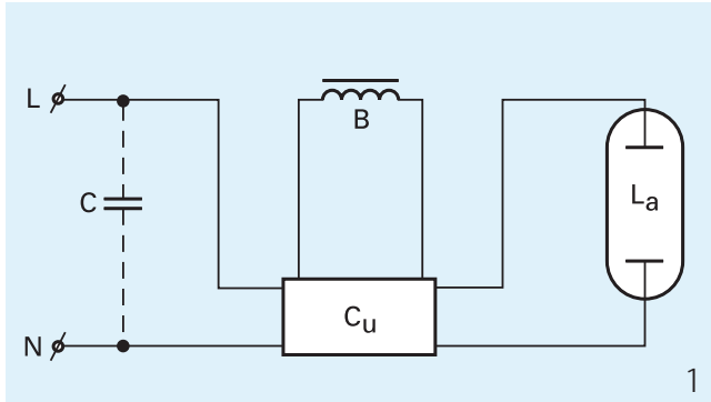
Schéma de câblage 1
