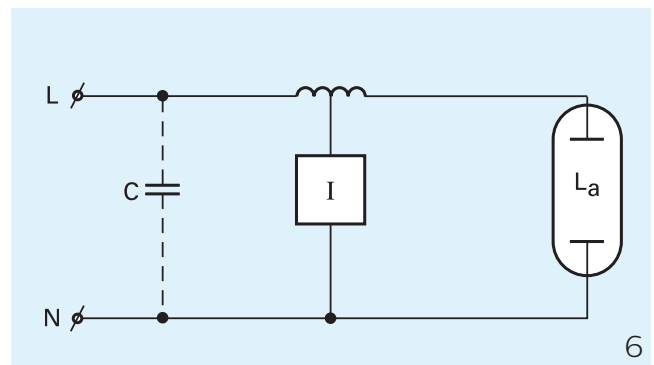
Schéma de câblage 6
