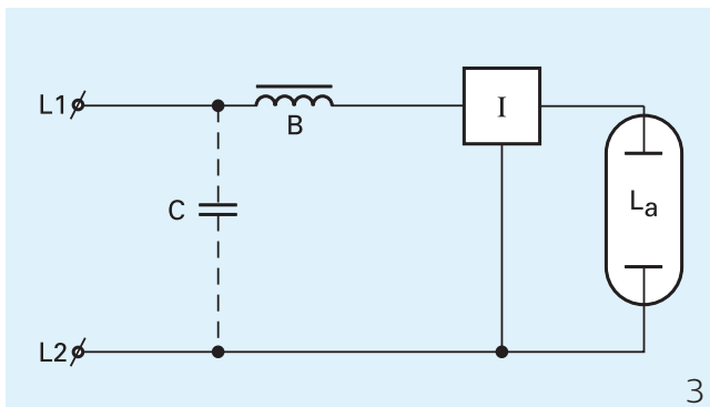
Schéma de câblage 3
