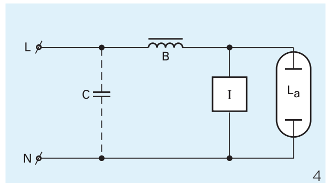
Schéma de câblage 4
