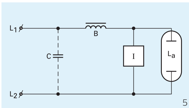
Schéma de câblage 5
