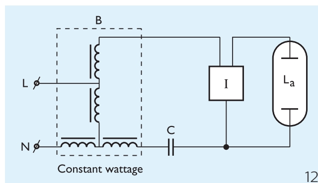
Schéma de câblage 12
