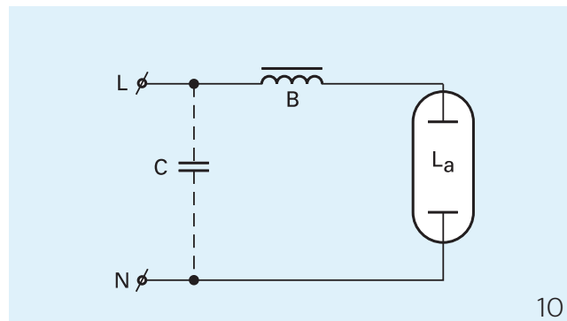
Schéma de câblage 10
