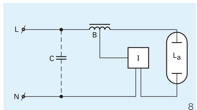
Schéma de câblage 8
