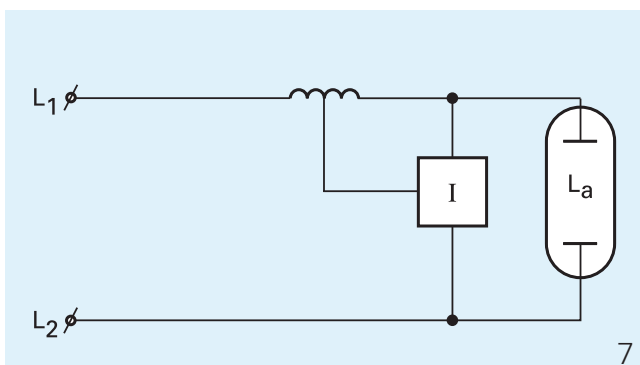
Schéma de câblage 7
