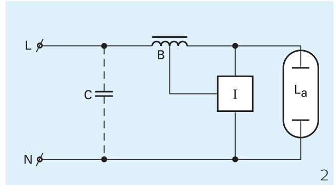
Schéma de câblage 2
