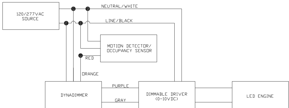
SCHEMA DE CÂBLAGE POUR MRO AVEC DYNADIMMER
