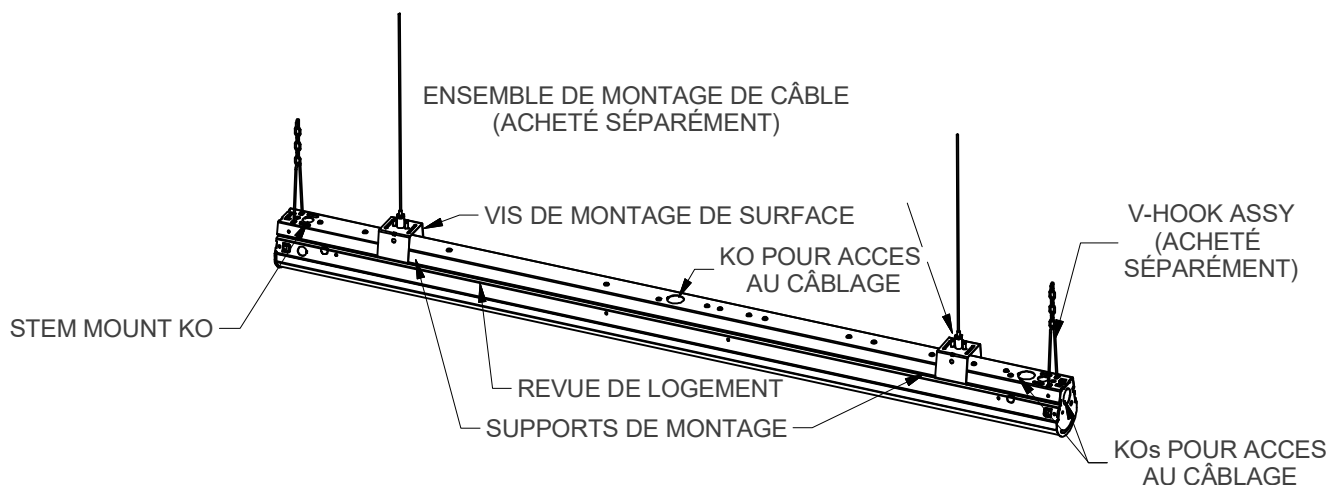
FIG 1 CONFIGURATION AUTONOME
