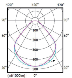
(cd/1000lm) 0° 90-270° SP402P, direkt, quadratisch
