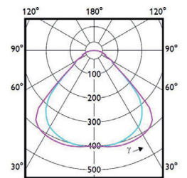
(cd/1000lm) 0° 90-270° SP402P, direkt, Langfeld
