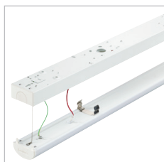
Für einfache Montage wird das Rückteil vom Vorderteil getrennt
