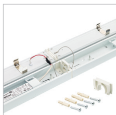
Lückenlose Verbindung mit Schnellverbinder ermöglicht ein durchgehendes Lichtband.
