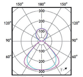
(cd/1000lm) 0° 90-270° SP402P, direkt-indirekt
