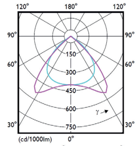
Breitstrahlende Optik (WB)
