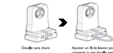
La figure montre comment modifier une douille sans shunt à une douille avec shunt à l'aide d'un fil de liaison.
