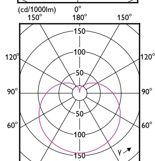
(cd/1000lm) 0°
