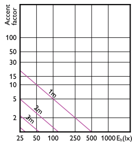
Accent Diagram - CoreProLEDspot D 4.3-60W R50 E14 827 36D
