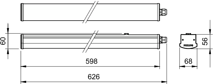
Σχεδιάγραμμα διαστάσεων
