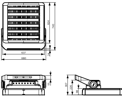
BVP621/BVP622/EVP622 SportsStar
