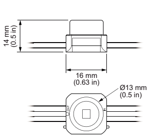
BGC482 50 4000K CLDM4 BK
