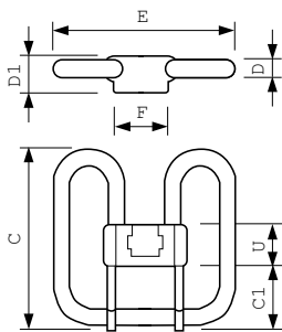
PL-Q 16W/830/2P
