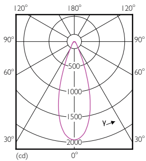
10-75W E26 PAR30L 40D 827 2700K
