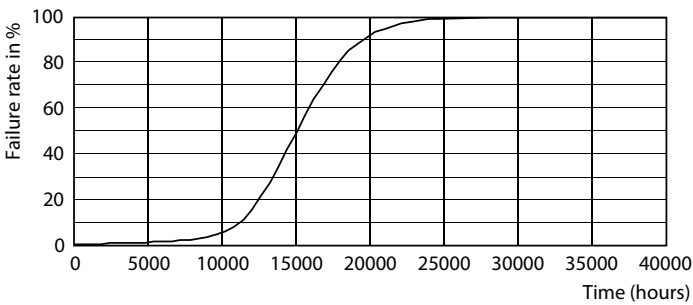
Life Expectancy Diagram - CLA LEDLuster D 5-32W P45 E14 822 GOLD
