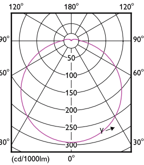
Light Distribution Diagram - 16UFO/LED/865/FR/P/ND 6/1FB
