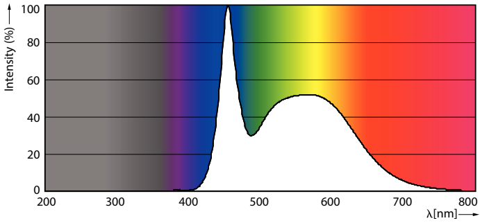
Spectral Power Distribution Colour - 16UFO/LED/865/FR/P/ND 6/1FB
