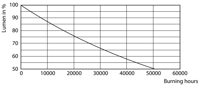
Lumen Maintenance Diagram - 5A19/MAS/927-22/FR/P/E26/T20 6/1CT
