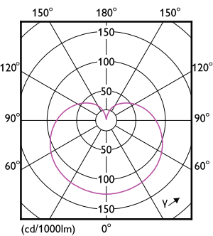
Light Distribution Diagram - 5A19/MAS/927-22/FR/P/E26/T20 6/1CT
