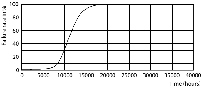
Life Expectancy Diagram - 9BR30/LED/827/FR/P/ND 4/3CT
