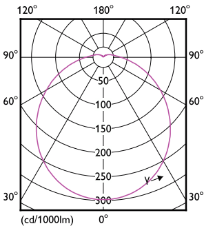
Light Distribution Diagram - 9BR30/LED/827/FR/P/ND 4/3CT
