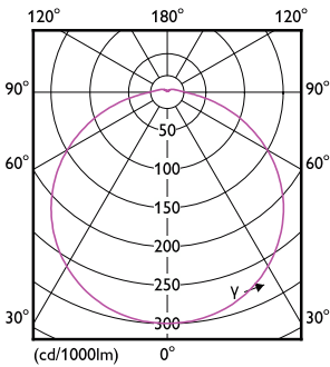
Light Distribution Diagram - 26UFO/PER/865/FR/P/E26/ND 4/1PF
