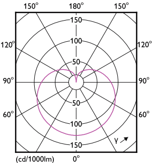
Light Distribution Diagram - 5A19/COR/927/FR/P/E26/DIM/T20 6/1CT
