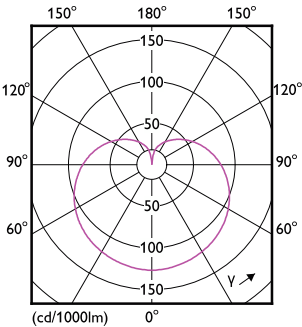
Light Distribution Diagram - 8.8A19/COR/927/FR/P/E26/DIM/T20 6/1CT
