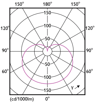
Light Distribution Diagram - 12.2A19/COR/950/FR/P/E26/DIM/T20 6/1CT
