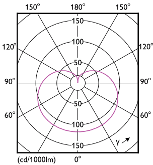
Light Distribution Diagram - 29A21/PER/850/FR/P/E26/D/HO 4/1PF
