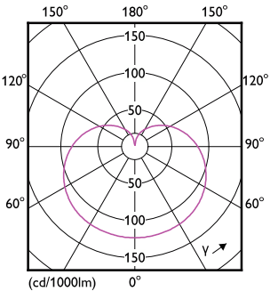
Light Distribution Diagram - 12.2A19/COR/927/FR/P/E26/DIM/T20 6/1CT
