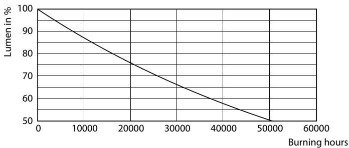
Lumen Maintenance Diagram - 12.2A19/COR/927/FR/P/E26/DIM/T20 6/1CT
