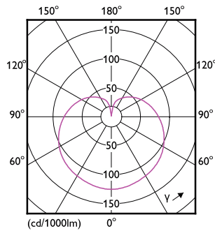
Light Distribution Diagram - LEDLuster 5W P45 2700K E27 ND FR AU 2CT
