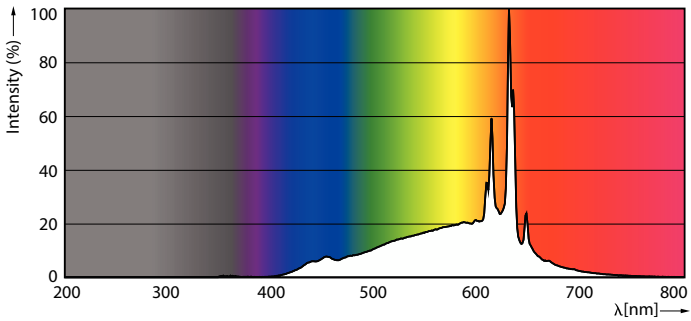
Spectral Power Distribution Colour - 5B11/PER/CRI95WG/FR/G/E12/WGD 1CT T20
