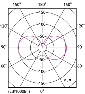
Light Distribution Diagram - 5B11/PER/CRI95WG/FR/G/E12/WGD 1CT T20
