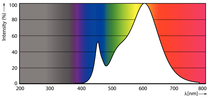
Spectral Power Distribution Colour - LEDSpot 35W DS ND GU10 60D 1CT/6 AU
