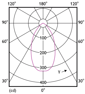
Light Distribution Diagram - LEDSpot 35W DS ND GU10 60D 1CT/6 AU
