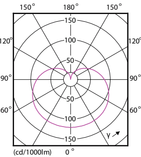
Light Distribution Diagram - 14A19/COR/927/FR/P/E26/DIM/T20 6/1CT
