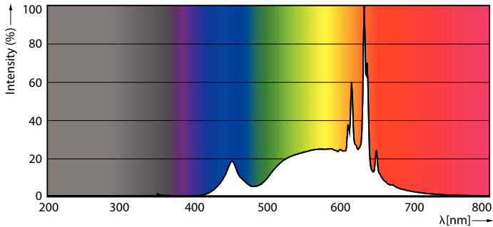
Spectral Power Distribution Colour - 14A19/COR/930/FR/P/E26/DIM/T20 6/1CT
