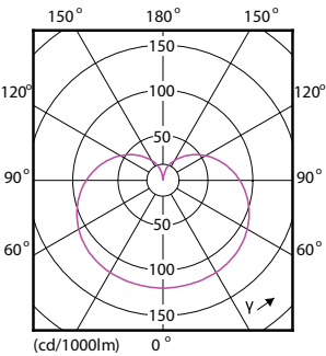
Light Distribution Diagram - 14A19/COR/930/FR/P/E26/DIM/T20 6/1CT
