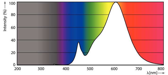
Spectral Power Distribution Colour - LEDBulb 9W B22 DS FR DIM 1PF/6 AU
