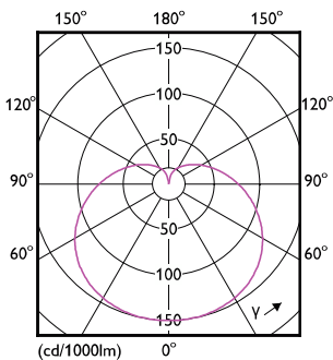
Light Distribution Diagram - LEDBulb 9W B22 DS FR DIM 1PF/6 AU
