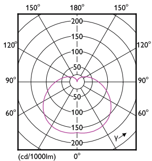
Light Distribution Diagram - LEDBulb 14W B22 DS FR DIM 1PF/6 AU
