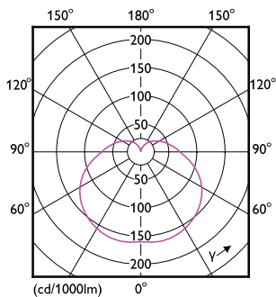
Light Distribution Diagram - LEDStick 10W B22 DS FR DIM 1PF/6 AU
