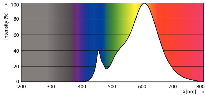
Spectral Power Distribution Colour - LEDStick 10W B22 DS FR DIM 1PF/6 AU
