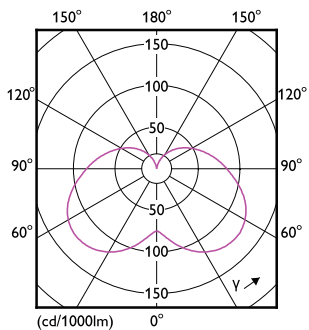
Light Distribution Diagram - LEDStick 14W E27 DS FR DIM 1PF/6 AU
