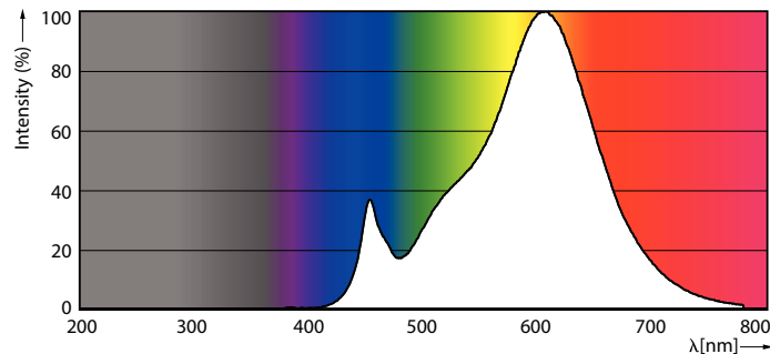
Spectral Power Distribution Colour - LEDstick 14W B22 DS FR DIM 1PF/6 AU
