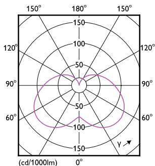
Light Distribution Diagram - LEDstick 14W B22 DS FR DIM 1PF/6 AU
