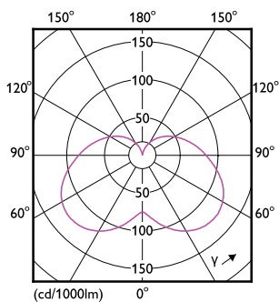
Light Distribution Diagram - LEDStick 14W B22 DS FR DIM 1PF/6 AU
