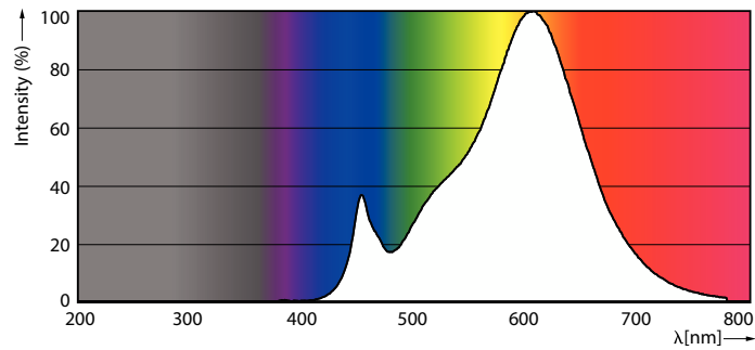
Spectral Power Distribution Colour - LEDStick 14W B22 DS FR DIM 1PF/6 AU
