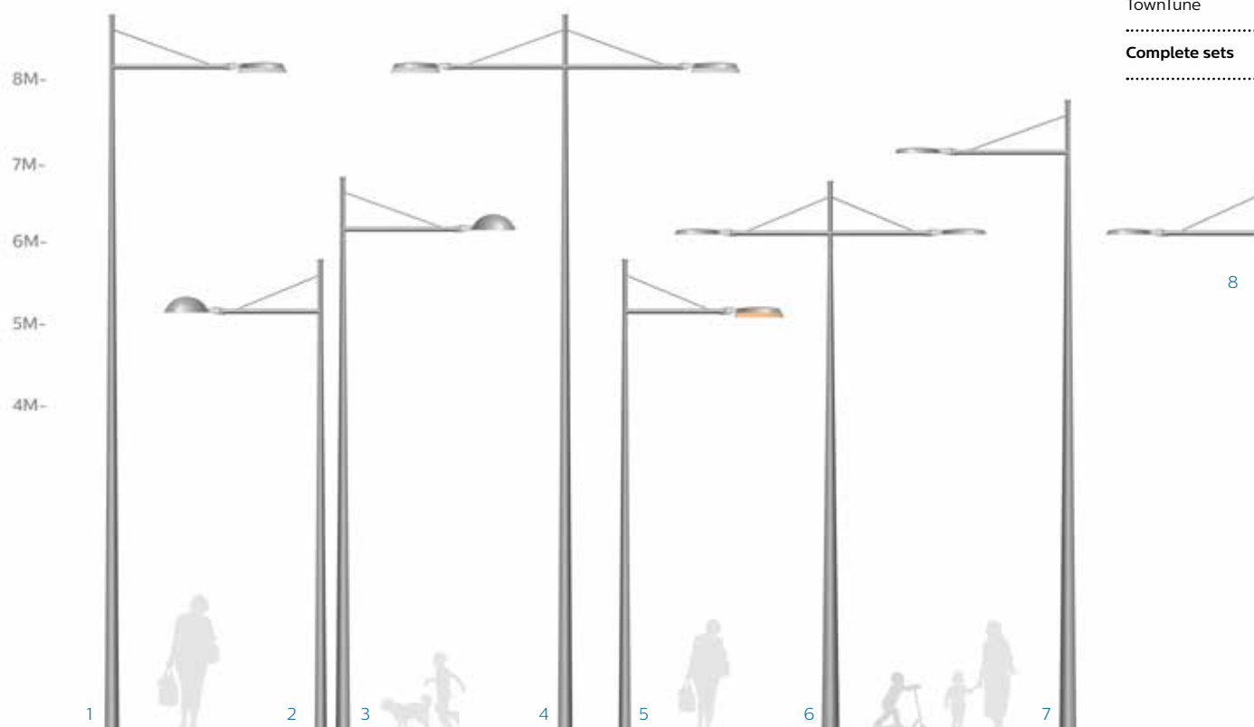
1-4. Accante-mast 8 m + Caravelle Low-uthouder S1400 + TownTune-armatuur BDP266-60 met ring 2. Accante-mast 5 m + Caravelle Low-uthouder S1200 + TownTune-armatuur BDP268-60 3. Accante-mast 6 m + Caravelle Low-uthouder S1400 + TownTune-armatuur BDP268-60 met ring 5. Accante-mast 5 m + Caravelle Low-uthouder S1200 + TownTune-armatuur BDP266-60 met ring 6. Accante-mast 6 m + Caravelle Low-uthouder S1200 + TownTune-armatuur BDP265-60 7. Accante-mast 7 m + Caravelle Low-uthouder S1400 + TownTune-armatuur BDP265-60 8. Caravelle Low-wandverlichting S1200 + TownTune-armatuur BDP265-60
