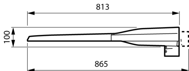
LumiStreet gen2 PRO groot
