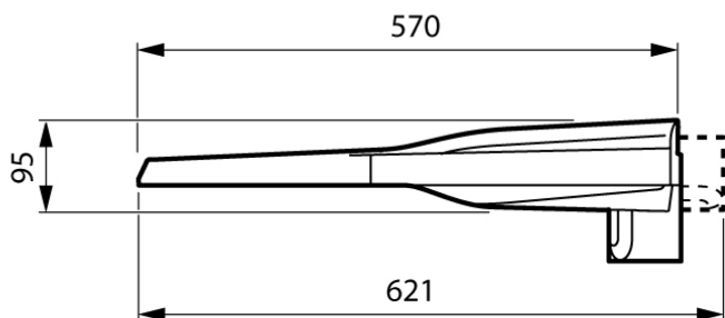
LumiStreet gen2 PRO mini
