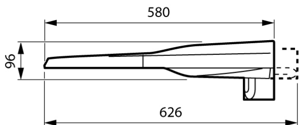
LumiStreet gen2 PRO middelgroot
