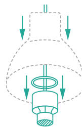
7 Abaissez l'anneau de montage et la nouvelle vasque décorative : ils se positionnent automatiquement !
