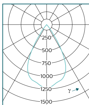
CustomCreate PT520T LED27S/830 VWB Faisceau très extensif
