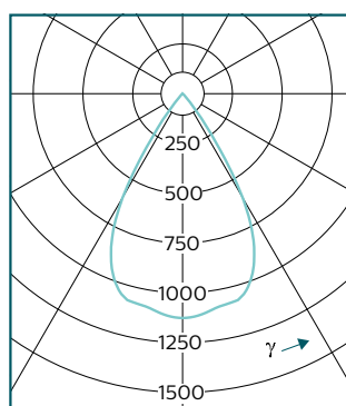
CustomCreate PT520T LED65S/830 VWB Faisceau très extensif
