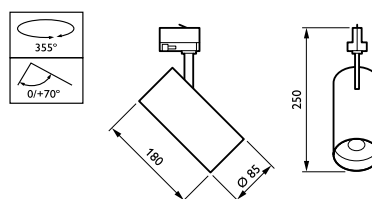
Dimensions en mm
