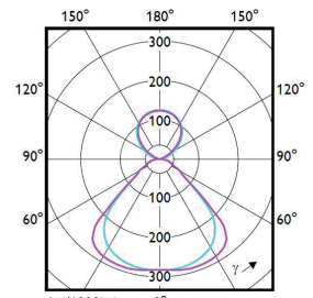
(cd/1000lm) 0° 90-270° SP402P, direkt-indirekt
