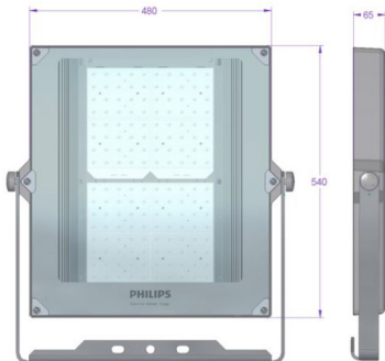
BVP140 Mått i mm
