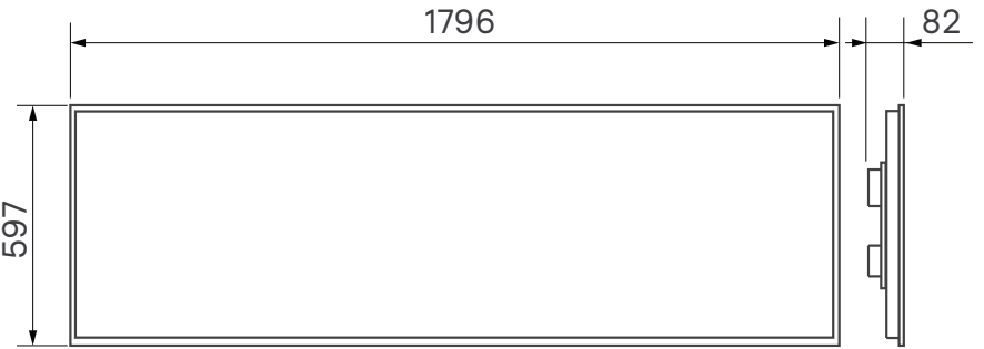
Mitat millimetreinä
