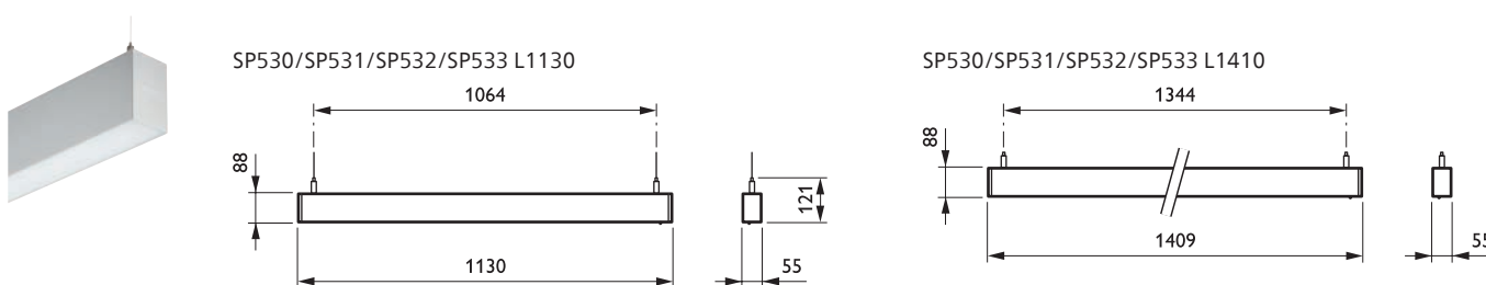
Anturilla varustetut valaisimet, L+40 mm
