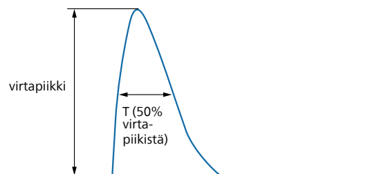
Syöksyvirta graafisesti esitettynä
