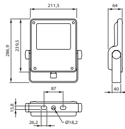
BVP611 - Dimensions en mm
