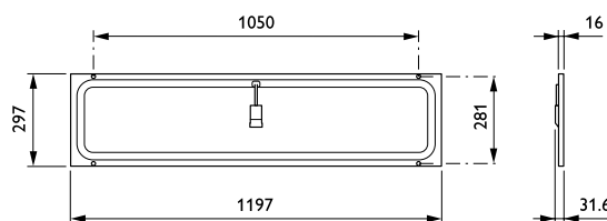
Version 300 x 1 200 - Dimensions en mm
