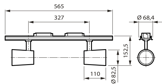
Version ST210Y double spots pour CoreLine Trunking - Dimensions en mm
