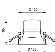
Version cardanique Compact (RS771B)
