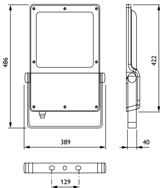
BVP130 - Dimensions en mm
