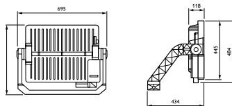
BVP518 (2 modules) avec driver déporté
