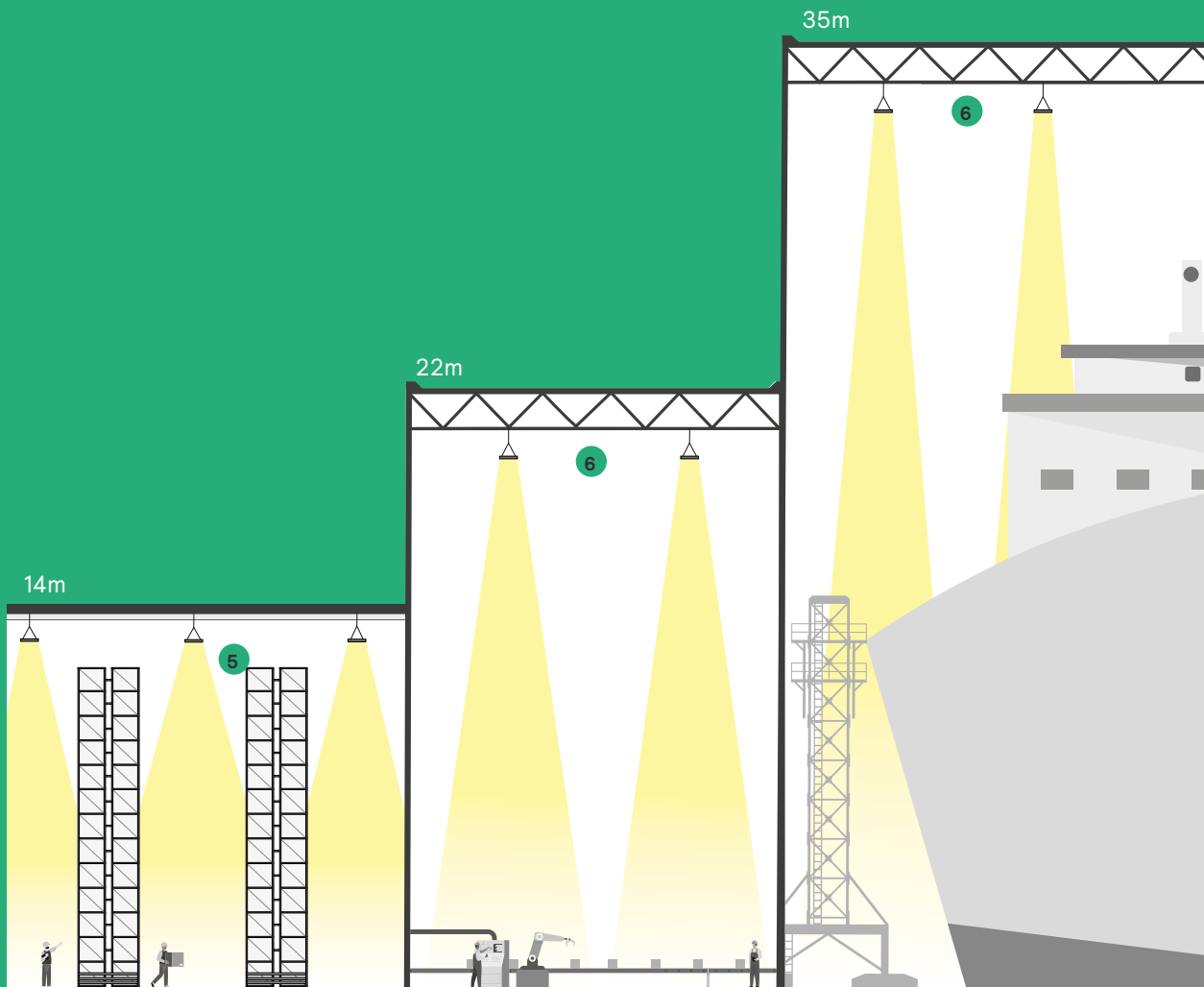
5 High rack optic (HRO) Hauteur d'installation >12m
