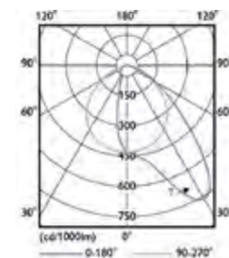
SM534C, asymmetrisch
