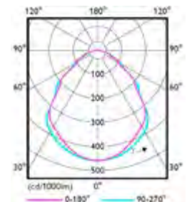
SM402C, quadratisch
