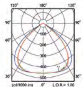
mittelbreitstrahlend (MB)
