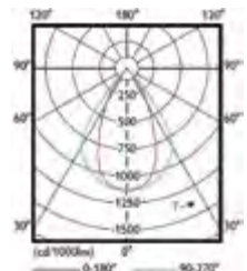
Engstrahlend (NB)
