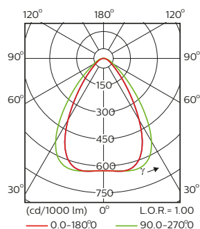
MB (Medium beam)
