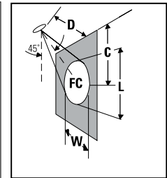
45° Aiming Angle
