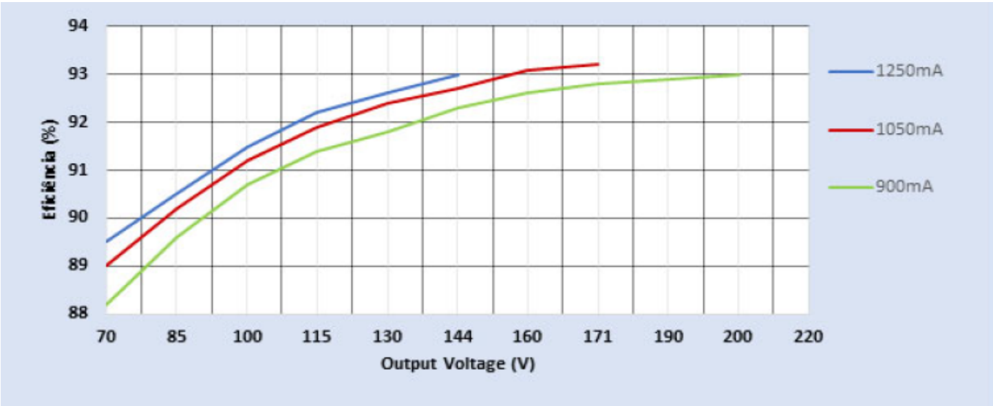
Eficiência Vs. Tensão de saída (Tensão de entrada em 277Vac)
