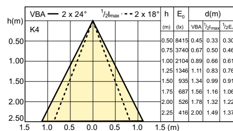
Beam diagram - CDM-Rm Elite Mini 20W/830 GX10 MR16 40D
