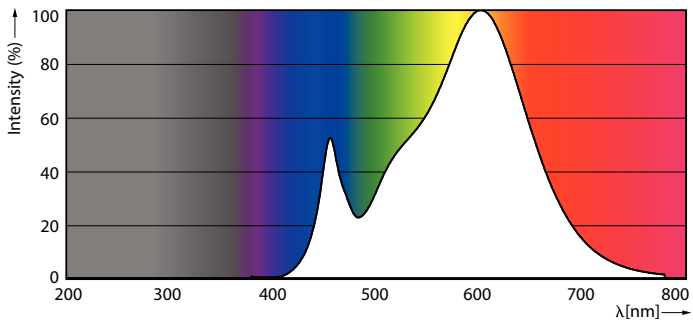
Spectral Power Distribution Colour - 16UFO/PER/830/FR/P/E26/ND 4/1PF
