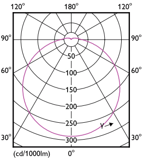
Light Distribution Diagram - 16UFO/PER/830/FR/P/E26/ND 4/1PF
