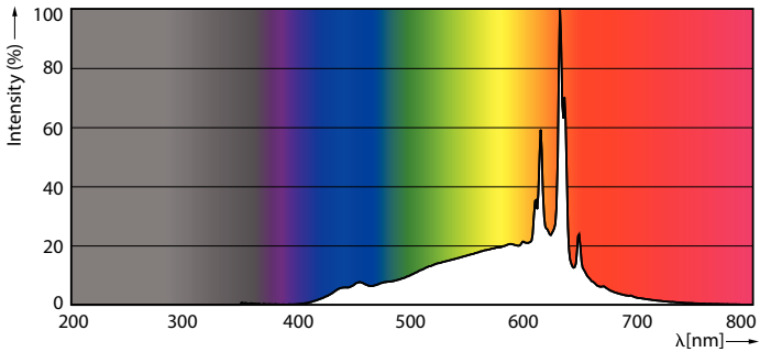
Spectral Power Distribution Colour - 5BA11/PER/CRI95WG/FR/G/E12/WGD 1CT T20
