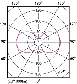
Light Distribution Diagram - 5BA11/PER/CRI95WG/FR/G/E12/WGD 1CT T20
