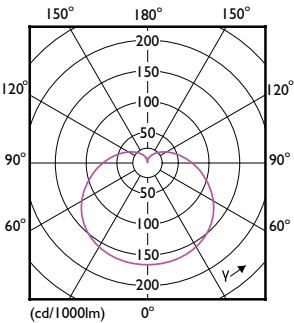
Light Distribution Diagram - LEDBulb 12W E27 930 230V 1PF/6 AU
